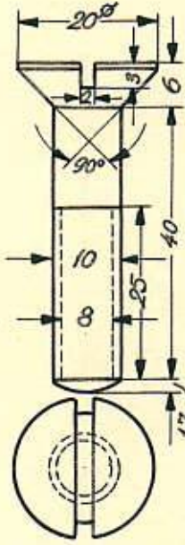
Senk, M 10 x 40, Din 87
