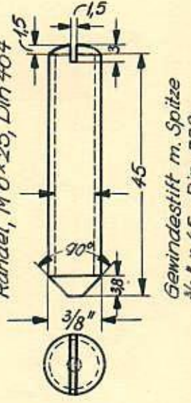
Rändel, M 6 x 25, Din 464
